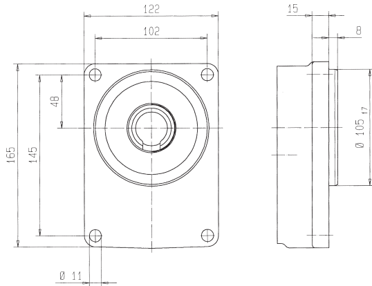
Rechteck-4-Loch-Flansch G nur KP 2
