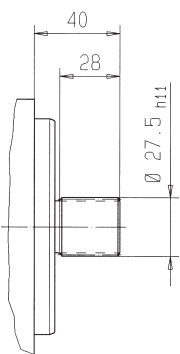
Wellenende W Zahnwellenprofil B 28 x 25 DIN 5482 z = 15, m = 1,75 450 Nm max
