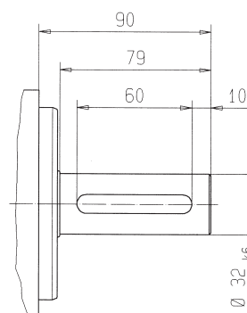
Wellenende Y Zylindrische Welle 550 Nm max
