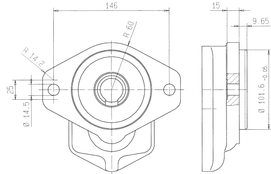
SAE-B-2-Loch-Flansch S
